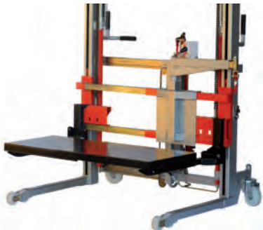
Art.-Nr. 302.206 mit ausziehbarer Platte Plattenmaße: Breite 640 - 1140 mm Tiefe 460 mm
