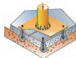
Zwischenplatte auf einem Stahlbetonboden / auf einer Stahlbetondecke (Mehrpreis auf Anfrage)
