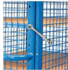
Bodenträger variabel einsetzbar, Teilung 100 mm
